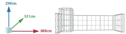
MODU-220
