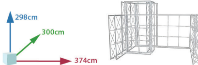
MODU-213
